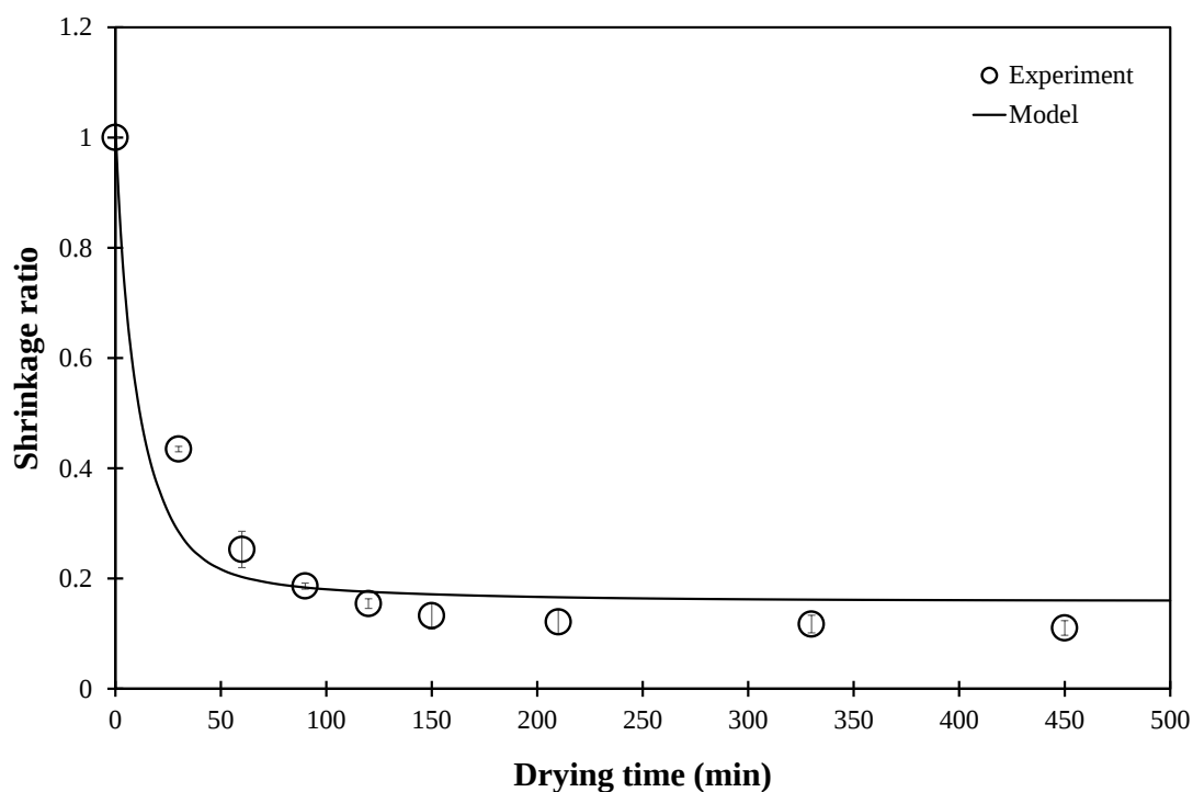
ภาพประกอบที่ 45 การเปลี่ยนอัตราส่วนการหดตัวที่ได้จากแบบจำลองที่อุณหภูมิ 80°C
