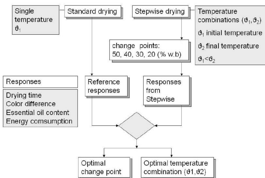
ภาพประกอบที่ 13 การเปรียบเทียบวิธีการอบแห้งแบบมาตรฐานและวิธีการอบแห้งแบบขั้นตอน (STEPWISE DRYING)
