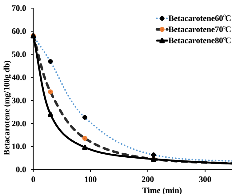
ภาพประกอบที่ 25 การเปรียบเทียบปริมาณเบต้าแคโรทีนเป็นฟังก์ชันของเวลาในการอบแห้งที่อุณหภูมิ 60, 70 และ 80°C
