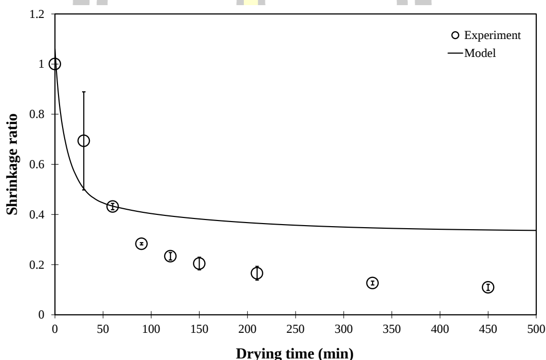
ภาพประกอบที่ 43 การเปลี่ยนอัตราส่วนการหดตัวที่ได้จากแบบจำลองที่อุณหภูมิ 60°C
