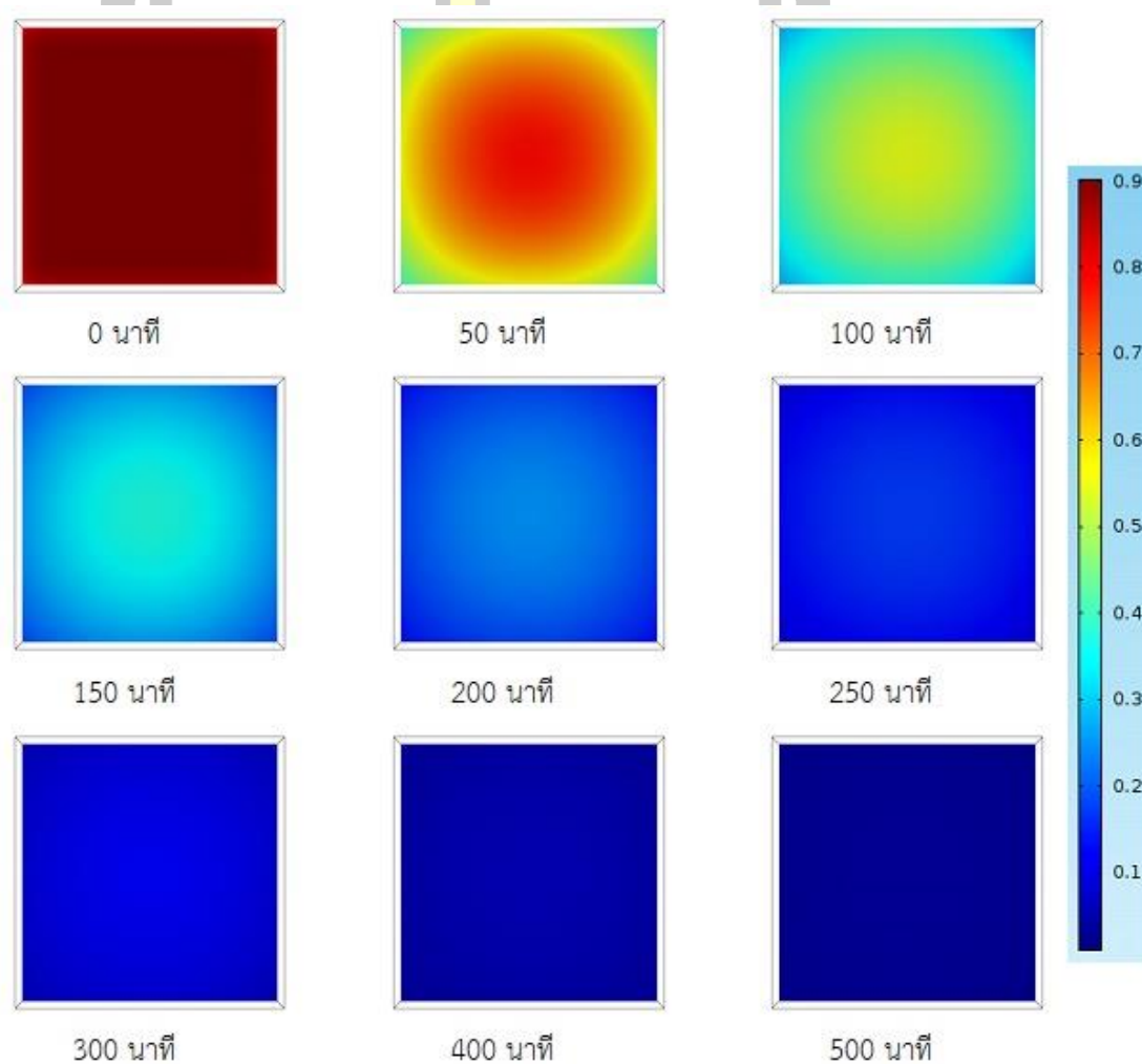
ภาพประกอบที่ 31 CONTOUR PLOTS แสดงการเปลี่ยนแปลงความชื้นที่เวลาอบแห้งต่างๆ ภายใต้ อุณหภูมิ 70^{\circ}\text{C}
