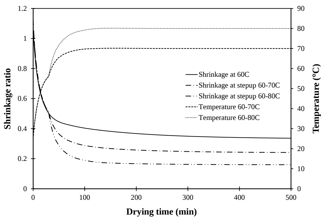
ภาพประกอบที่ 46 เปรียบเทียบผลการทำนายการหดตัวของกรอบแห้งแบบสองขั้นตอนในระยะเวลาอบแห้งที่ความแตกต่างกันแบบเพิ่มอุณหภูมิ 60 เป็น 70°C และ 60 เป็น 80°C กับค่าข้อมูลจากแบบจำลองที่อุณหภูมิการอบแห้งคงที่ 60°C
