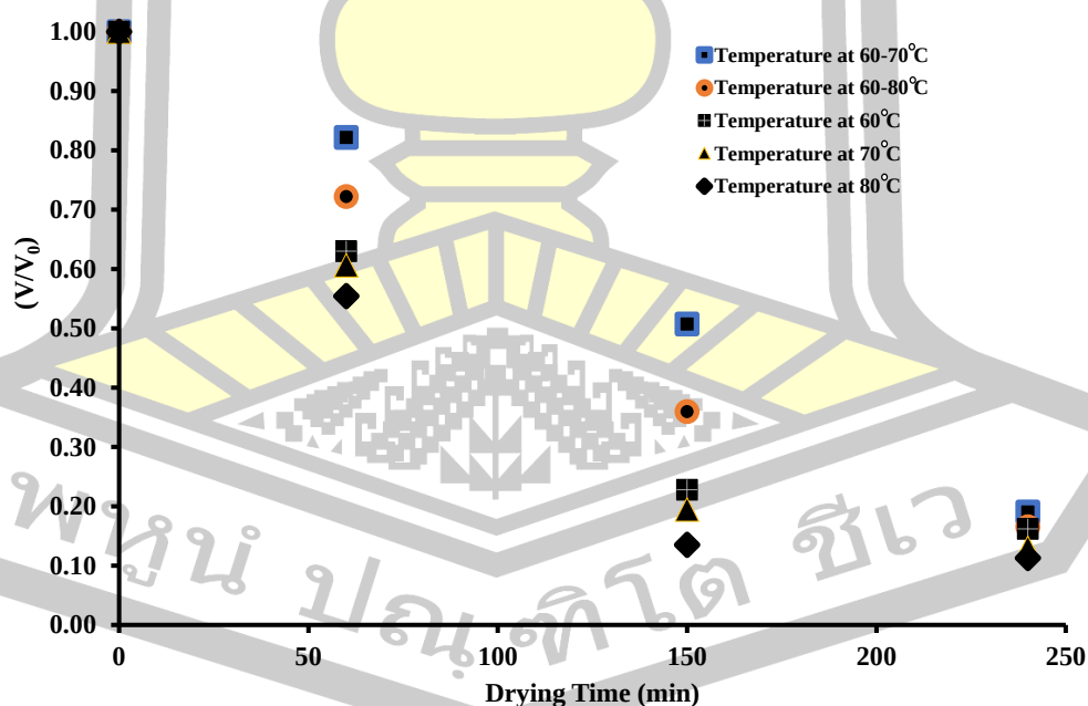
ภาพประกอบที่ 24 การเปรียบเทียบการหัตถ์ของแครอทอบแห้งแบบสองขั้นตอนแบบเพิ่ม อุณหภูมิ 60 เป็น 70^{\circ}\text{C} และ 60 เป็น 80^{\circ}\text{C} และการอบแห้งแบบคงที่
