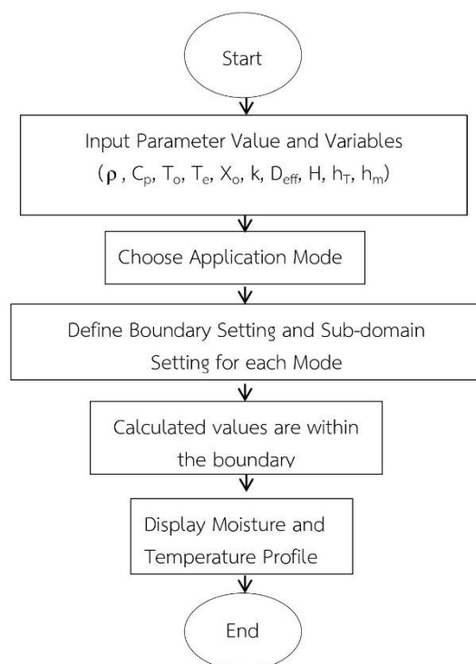
ภาพประกอบที่ 19 แผนภาพแสดงขั้นตอนการประมวลผลด้วยการจำลองทางคณิตศาสตร์ ที่มา: (Jomlapelatikul et al., 2016)
