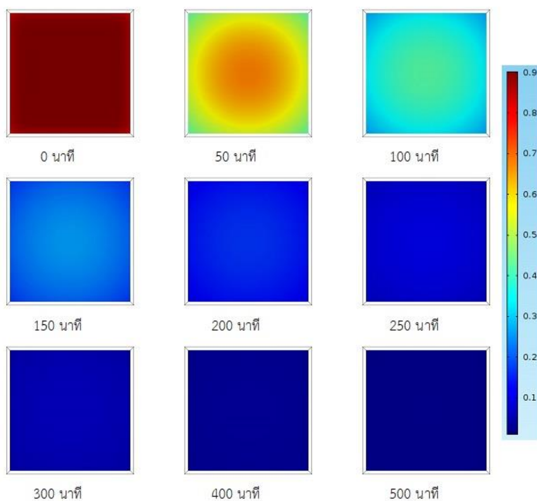
ภาพประกอบที่ 34 CONTOUR PLOTS แสดงการเปลี่ยนแปลงความชื้นที่เวลาอบแห้งต่างๆ ภายใต้ อุณหภูมิ 80^{\circ}\text{C}
