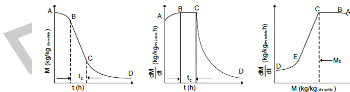
ภาพประกอบที่ 5 การลดลงของความชื้นวัสดุ
